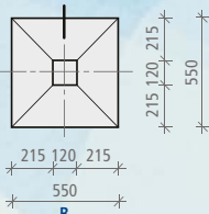
POHLAD ZDOLA
